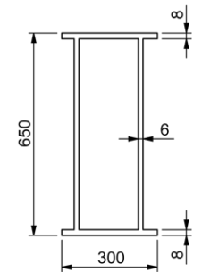
Mặt cắt dầm chính
